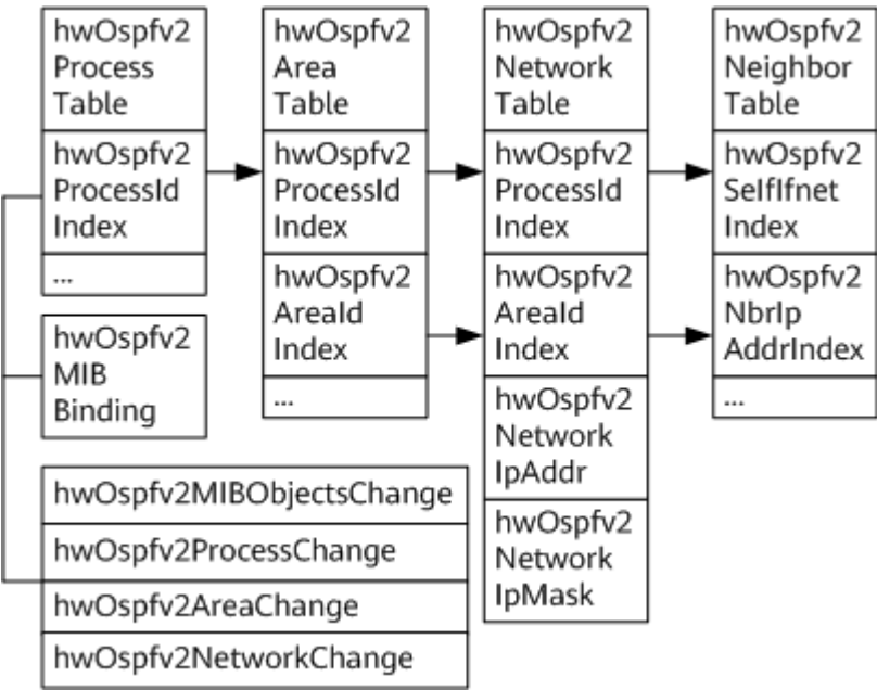
图 91-1 图 1 OSPF 策略表的表间关系图
